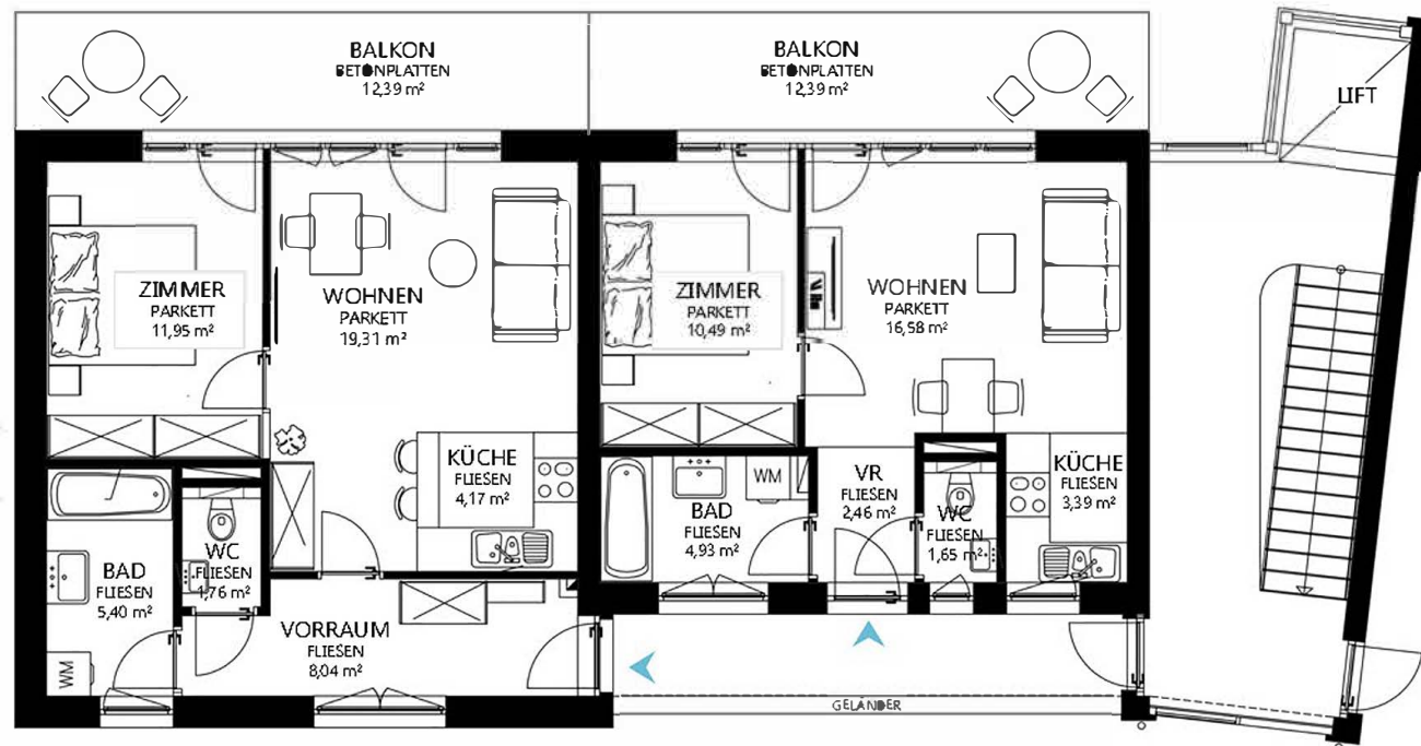
WFL 50,63 m 2 TOP 35
